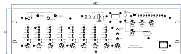
Fig1. Dimensioni per il montaggio
