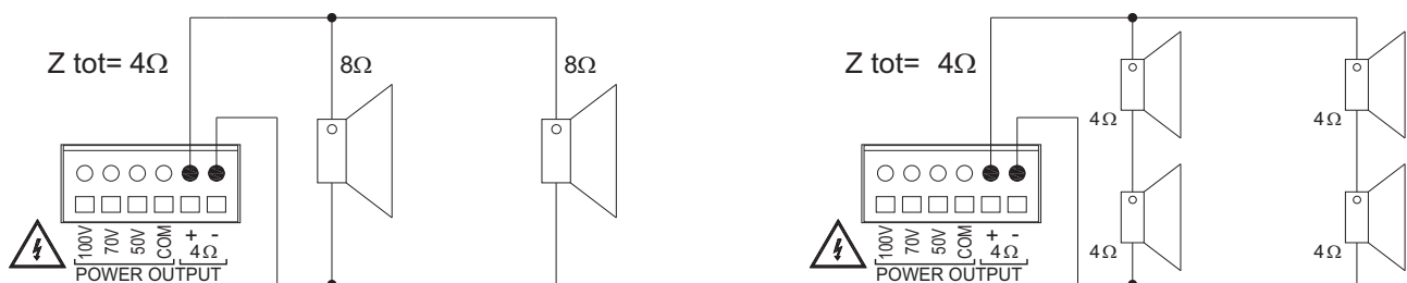
Fig3. Linee a impedenza costante
