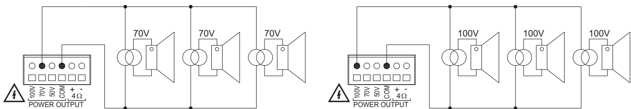
Fig2. Linee a tensione costante
